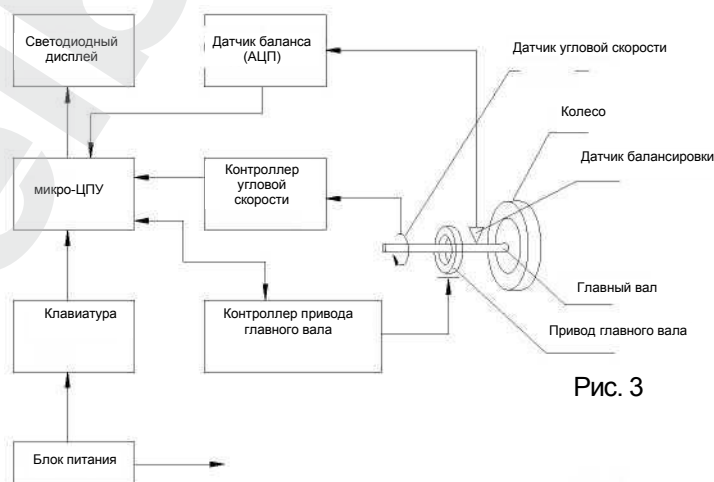
Рис. 3 Функциональная блок-схема балансировочного станка SB1930B
